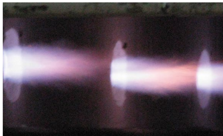
Flammen richtig und optimal eingestellter Brenner Flames correctly and optimum adjusted burner
